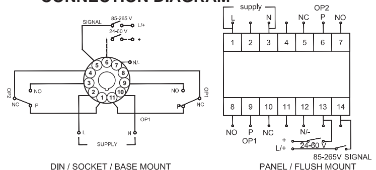
DIN / SOCKET / BASE MOUNT
